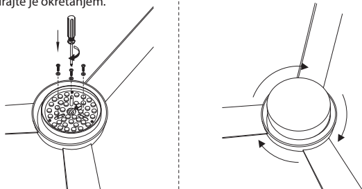
14. Fiksirajte modul šarafima koje ste izvadili iz držača i postavite buru, fiksirajte je okretanjem.
