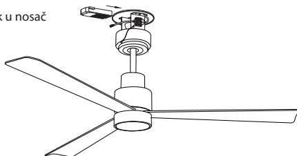
19. Priključite konektore u prijemnik i spojite uzemljenje
