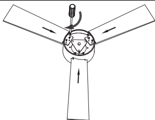
11. Šarafima pričvrstite lopatice za kućište motora
