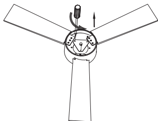
12. Odšarafite vijke koji fiksiraju LED modul i uklonite ga.
