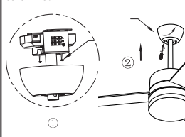
20. Fiksirajte dekorativni poklopac šarafima.
