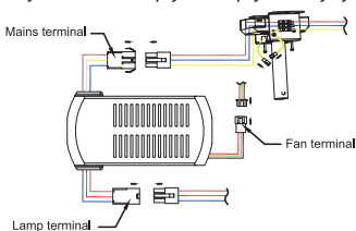
19. Priključite konektore u prijemnik i spojite uzemljenje.
