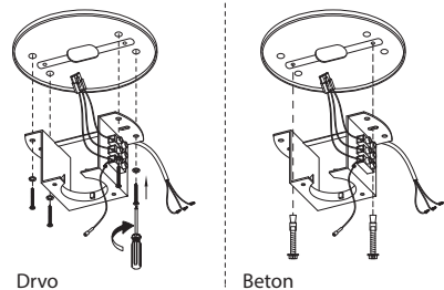
15. U zavisnosti od tipa podloge (drvo ili beton) fiksirajte nosač.
