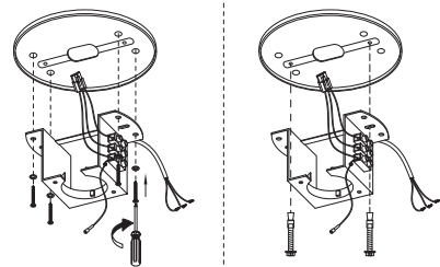
15. U zavisnosti od tipa podloge (drvo ili beton) fiksirajte nosač.
