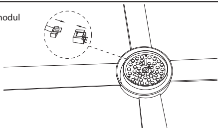
14. Fiksirajte modul šarafima koje ste izvadili iz držača i postavite buru, fiksirajte je okretanjem.
