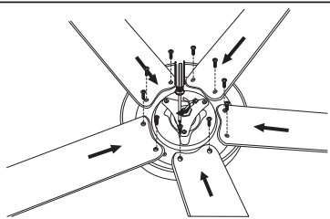
11. Šarafima pričvrstite lopatice za kućište motora
